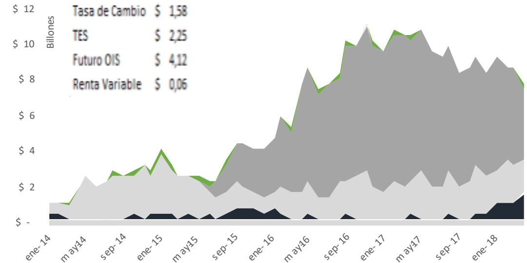
NOA por tipo de subyacente
